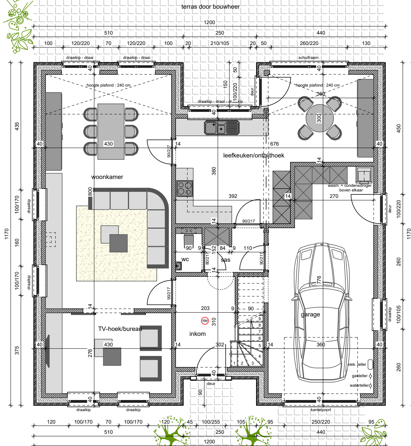
plan gelijkvloers
