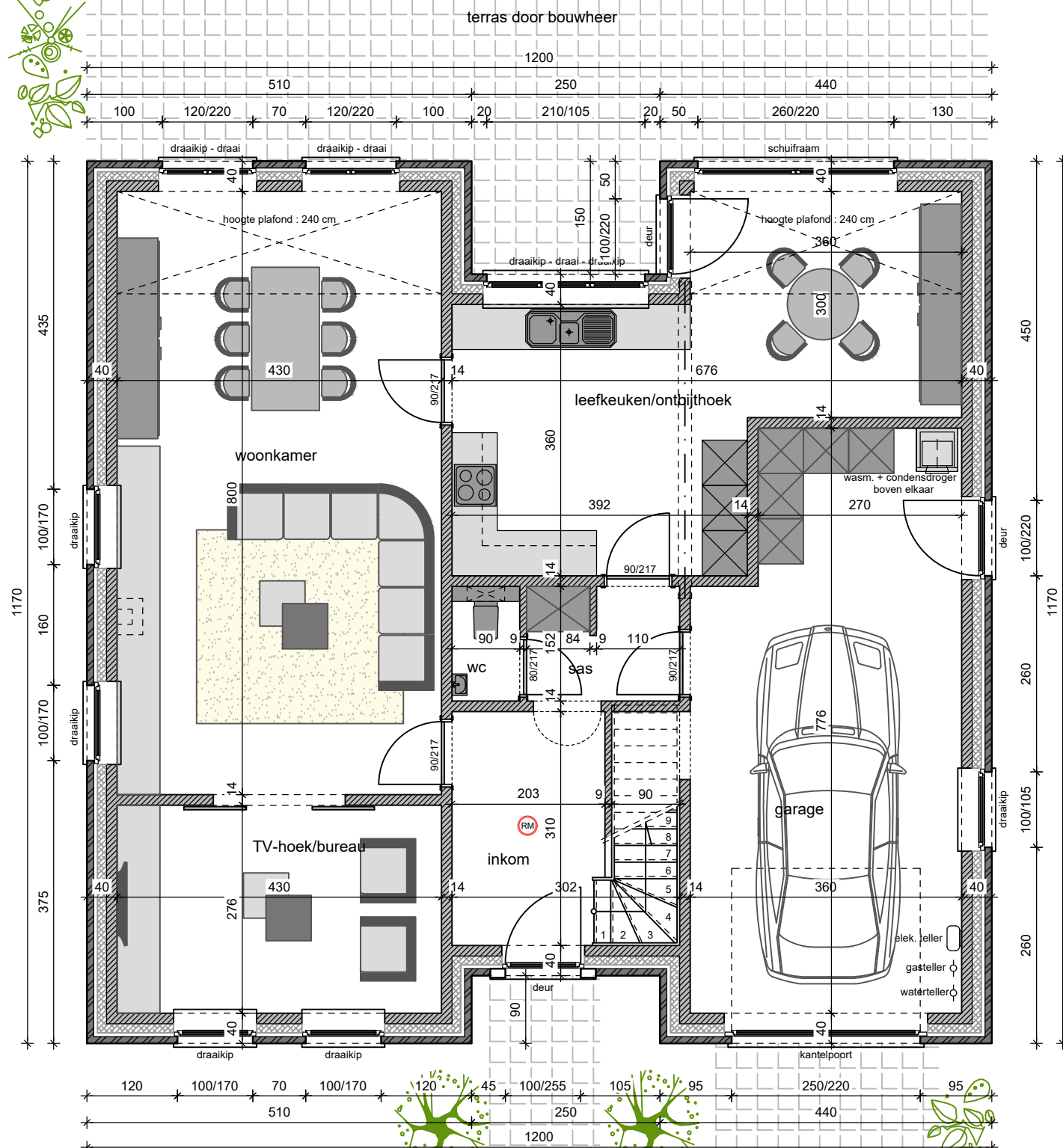
plan gelijkvloers
