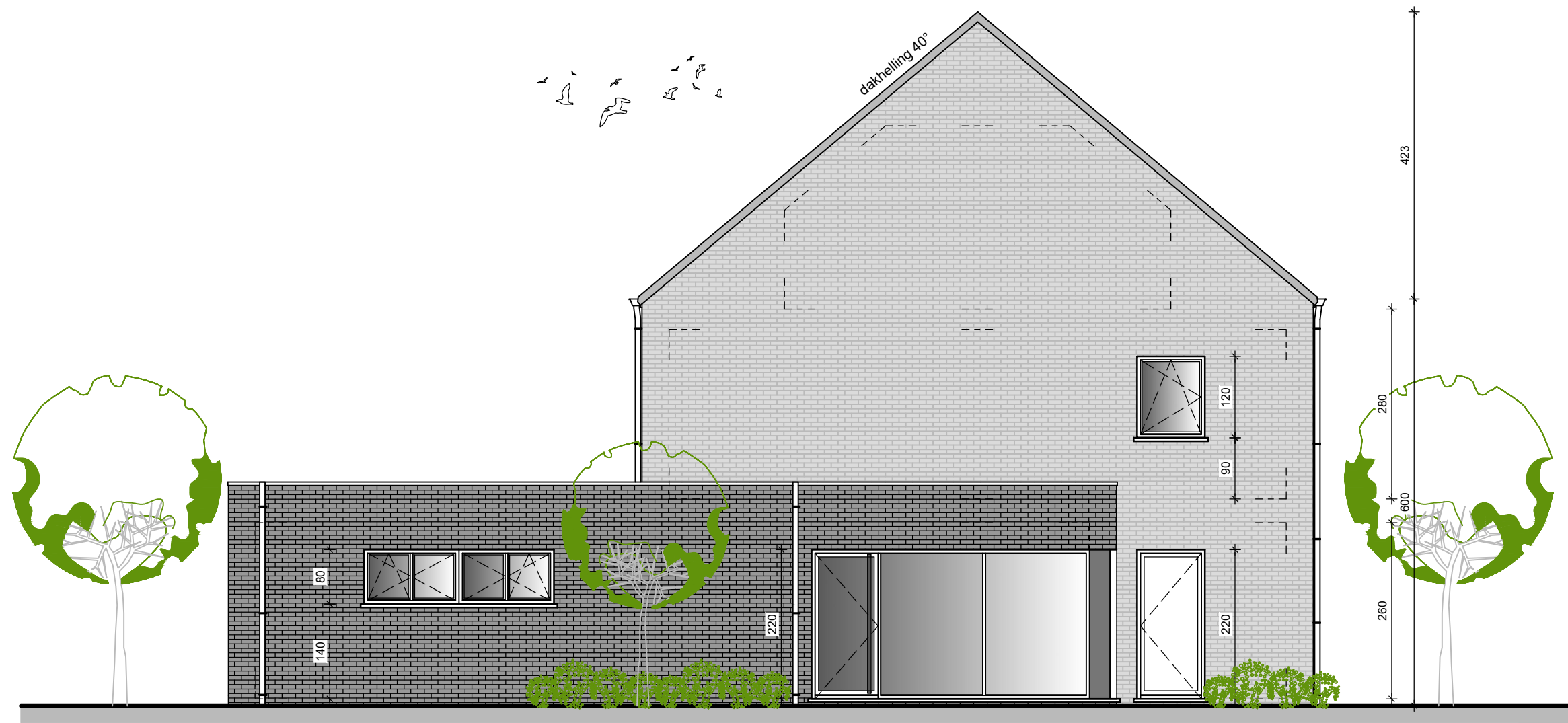
zijgevel rechts
