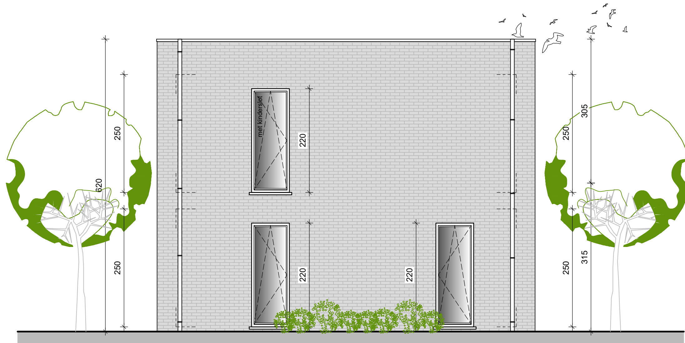
zijgevel rechts
