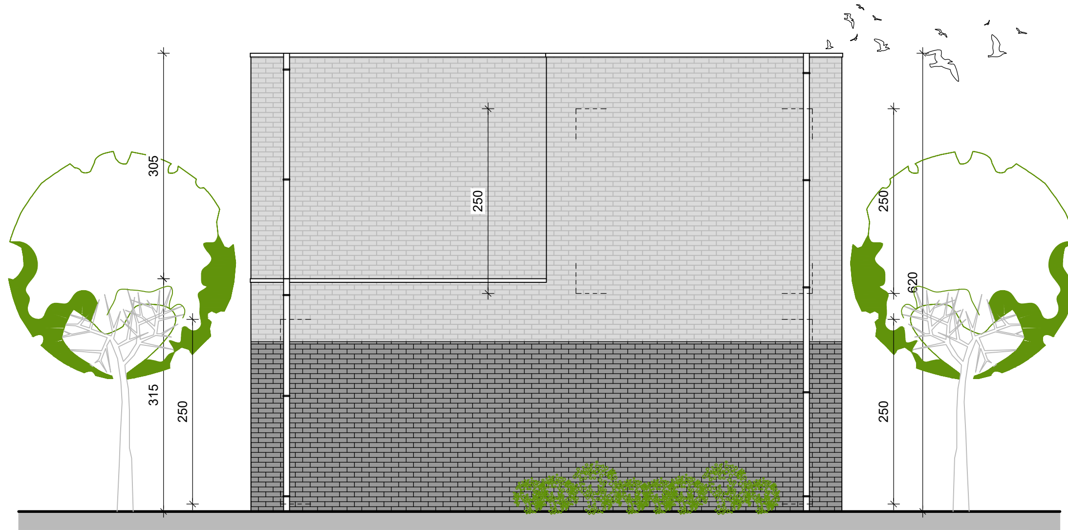
zijgevel links
